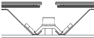
Abb. 5 Rückseite Modul „In-Joint“ Variante
