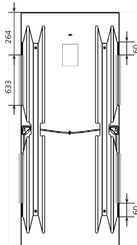
Abb. 5 Rückseite Modul „In-Joint“ Variante
