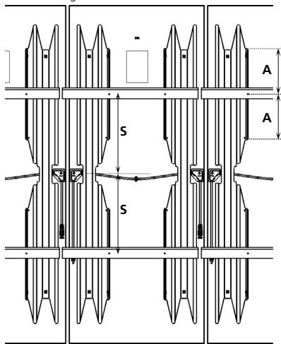
Abb. 3 Rückseite Modul „Hook-In“ Variante
