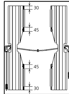
Abb. 6 Rückseite gekürzte Variante „Hook-In“ Montage bei einer Modullänge kleiner 1256 mm
